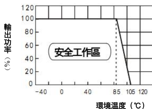
溫度曲綫圖
