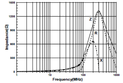
CMBM1608G301GSP
