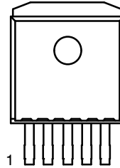
D 2 PAK-5
