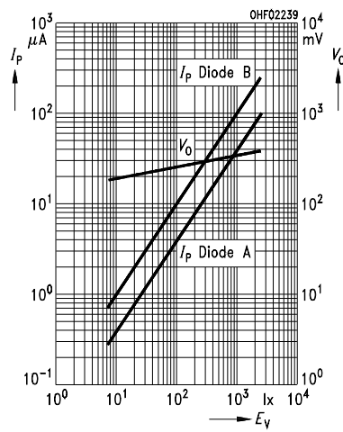
Photocurrent / Open-Circuit Voltage Fotostrom / Leerlaufspannung I_P (V_R = 5 \text{ V}) / V_O = f(E_V)
