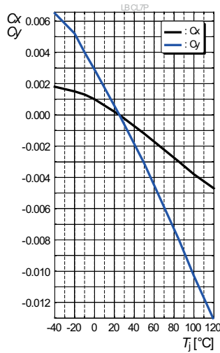
Chromaticity Coordinate Shift 5) page 20 Farbortverschiebung 5) Seite 20 C_x, C_y = f(T_j); I_F = 350 \text{ mA}
