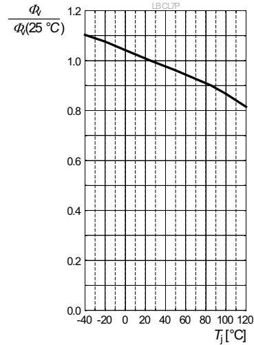
Relative Luminous Flux 5) page 20 Relative Lichtstrom 5) Seite 20 \Phi_V / \Phi_V(25^\circ\text{C}) = f(T_j); I_F = 350 \text{ mA}
