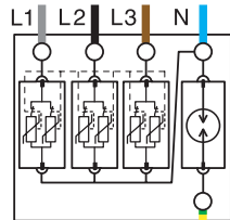
OVR T2 3N 40 275s P OVR T2 3N 70 275s P OVR T1+2 3N 7 275s P
