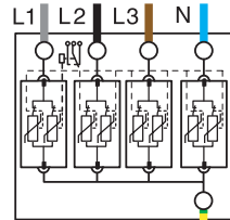
OVR T2 4L 40 275s P TS OVR T2 4L 70 275s P TS
