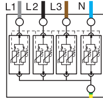
OVR T2 4L 40 275s P OVR T2 4L 70 275s P OVR T1+2 4L 7 275s P
