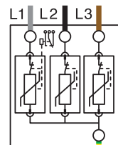
OVR T2 3L 15 275 P TS OVR T2 3L 40 275 P TS
