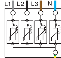
OVR T2 4L 15 275 P OVR T2 4L 40 275 P
