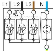
OVR T2 3N 40 275s P TS OVR T2 3N 70 275s P TS
