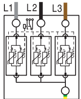
OVR T2 3L 40 275s P TS OVR T2 3L 70 275s P TS
