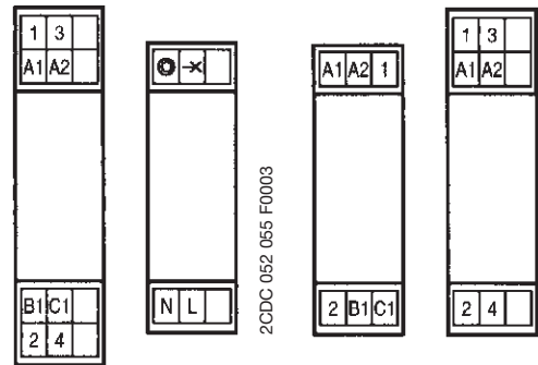
E 266 C E 262 C E 261-SRV E 261 E 261 C E 266 E 262
