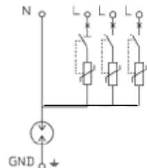
OVR Plus N3 20
