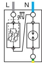
OVR T2 1N 40 275s P TS OVR T2 1N 70 275s P TS
