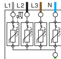
OVR T2 4L 15 275 P TS OVR T2 4L 40 275 P TS
