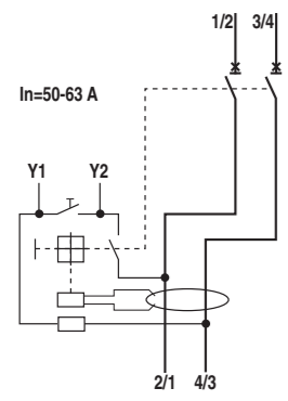
DS 204
