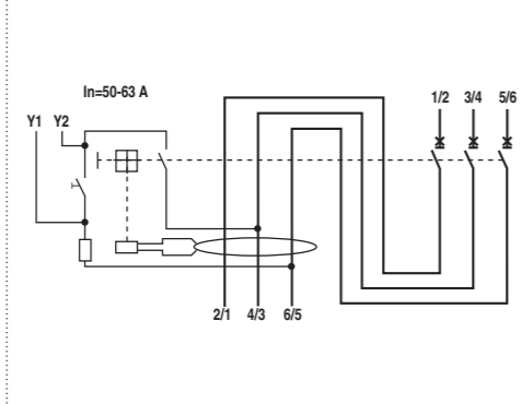
DS 203
