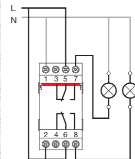
TWA-2
