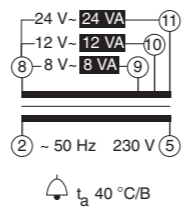
TS24/8-12-24
