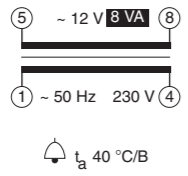
TS8/12 SW
