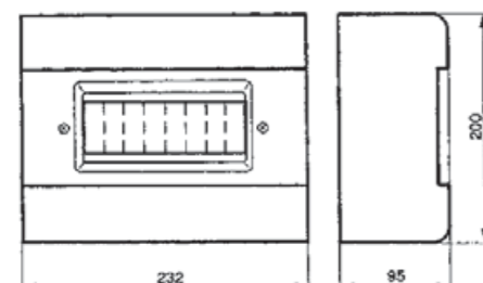
PCD 8 N
