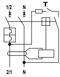
DS201
