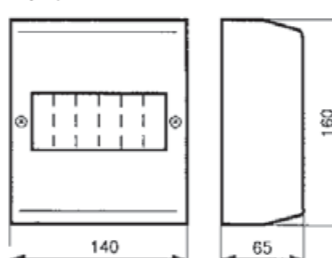
PCD 6 N
