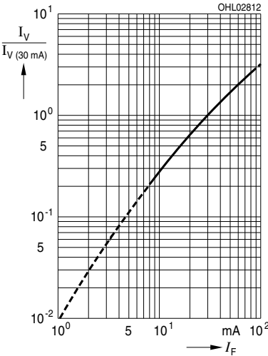
Relative Luminous Intensity 7) page 20, 8) page 20 Relative Lichtstärke 7) Seite 20, 8) Seite 20 I_V/I_V(30\text{ mA}) = f(I_F); T_S = 25\text{ }^\circ\text{C}
