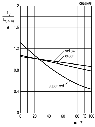
Relative Luminous Intensity 7) page 18 Relative Lichtstärke 7) Seite 18 I_V/I_V(25^\circ\text{C}) = f(T_j); I_F = 2\text{ mA}
