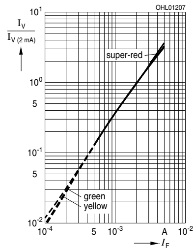
Relative Luminous Intensity 7) page 18, 8) page 18 Relative Lichtstärke 7) Seite 18, 8) Seite 18 I_V/I_V(2\text{ mA}) = f(I_F); T_S = 25^\circ\text{C}
