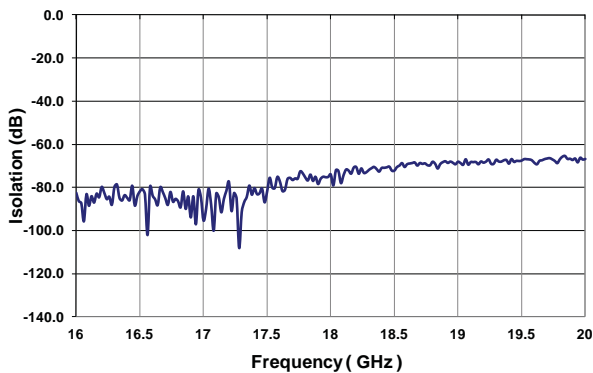
Isolation (16-20 GHz)
