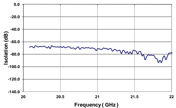
Isolation (20-22 GHz)
