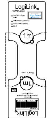
Label(48*150mm R=2mm)
