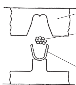
Obermatritze (Crimpstempel) Crimp indenter Abisolierter Leiter, in oder über der Leitercrimphülse positioniert Stripped wire in or above the conductor crimp barrel Offene Crimphülse mit geschrägten Außenflanken Open crimp barrel with chamfered outer flanks
