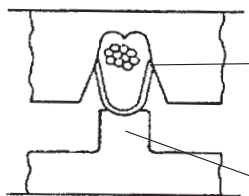
Die geschrägten Außenflanken dienen der besseren Führung der Crimphülse in der Obermatritze als auch dem besseren Einrollen der Crimphülsenflanken Better guidance of the crimp barrel in the crimp indenter by the chamfered outer flanks
