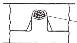
Die geschrägten Außenflanken dienen der besseren Führung der Crimphülse in der Obermatritze als auch dem besseren Einrollen der Crimphülsenflanken Better guidance of the crimp barrel in the crimp indenter by the chamfered outer flanks
