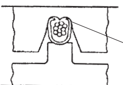
Untermatritze (Amboss) Crimp anvil Obermatritze und die sich einrollenden Crimphülsenflanken zwingen das abisolierte Leiterende in den Crimphülsenboden The indenter and the rolling up crimp flanks force the stripped conductor end into the base of the crimp barrel
