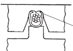
Obermatrize und die sich einrollenden Crimphülsenflanken zwingen das abisolierte Leiterende in den Crimphülsenboden
