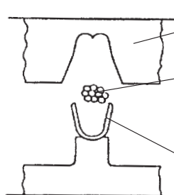
Obermatrize (Crimpstempel)
