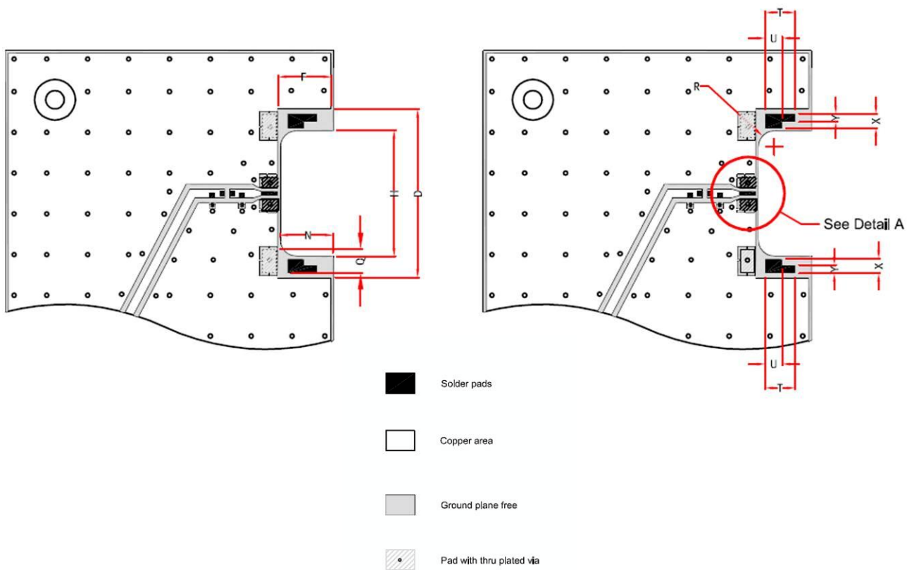
GPS Co-planar (Part No: A10137)
