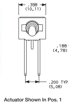
Actuator Shown In Pos. 1
