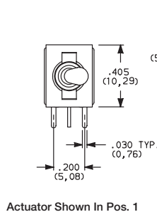
Actuator Shown In Pos. 1
