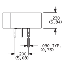
Actuator Shown In Pos. 1
