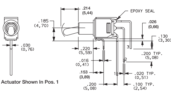
Actuator Shown In Pos. 1
