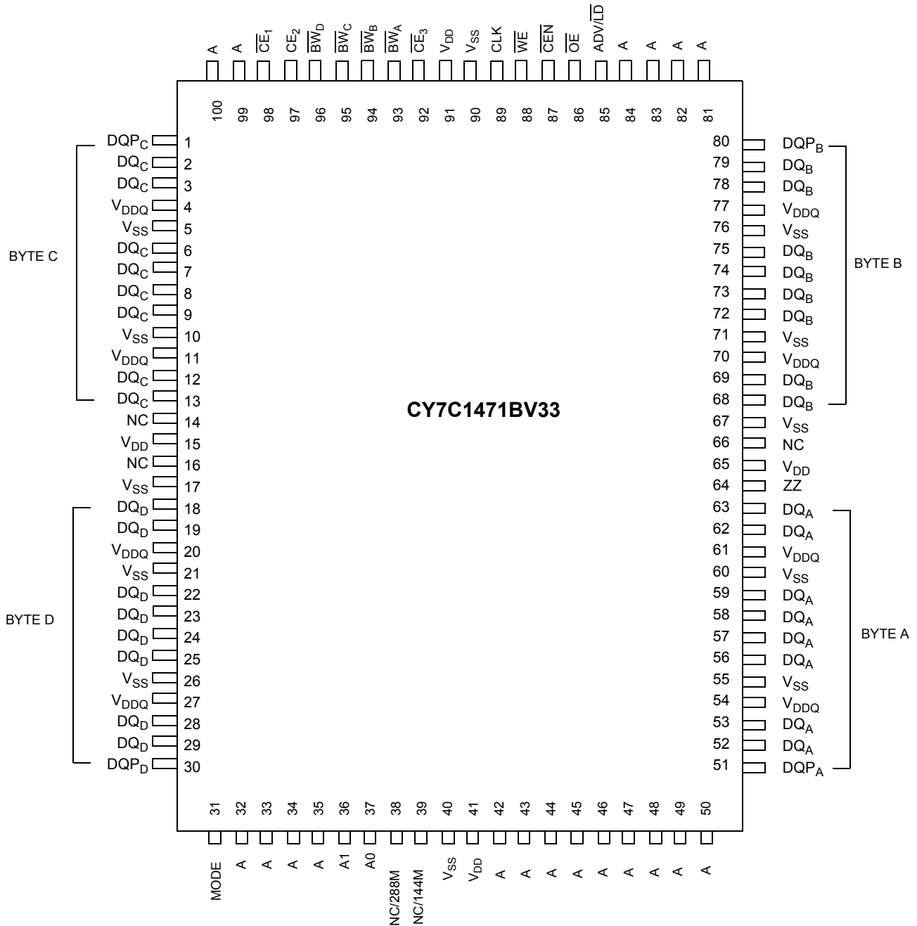
CY7C1471BV33 (2 M × 36)
