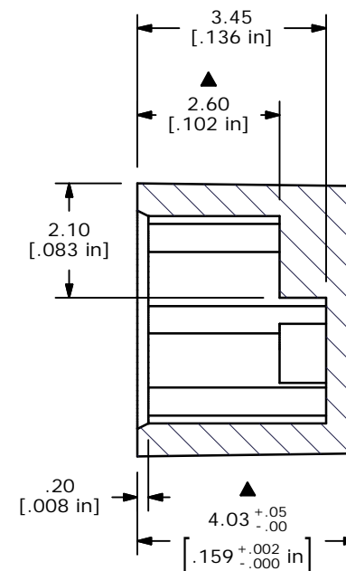
SECTION A-A SCALE 8 : 1
