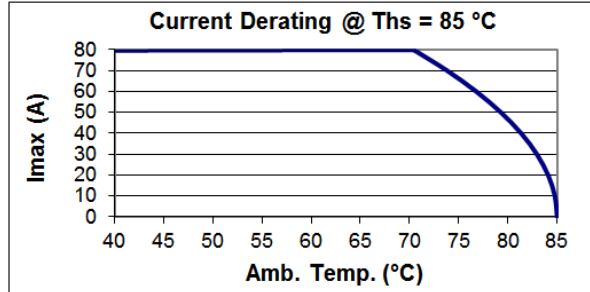
B25620D1617K101
