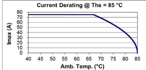
B25623B1447K204
