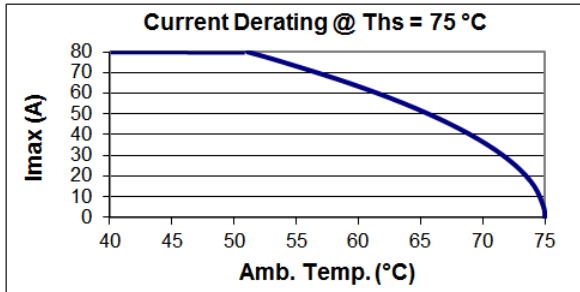
B25620B1617K103
