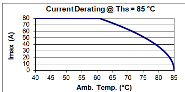
B25620B1487K101
