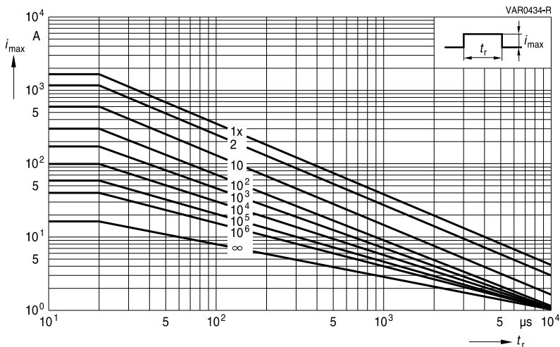
SIOV-S07K130 ... K320E2
