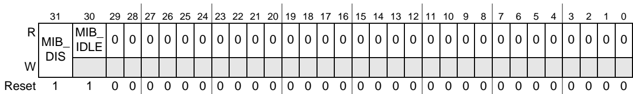
Figure 17-9. MIB Control Register (MIBC)
