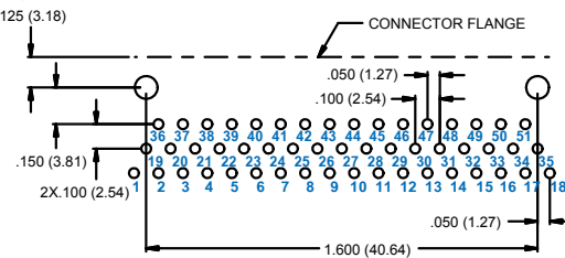
51 SOCKET M83513/20-G
