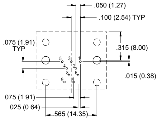
9 SOCKET
