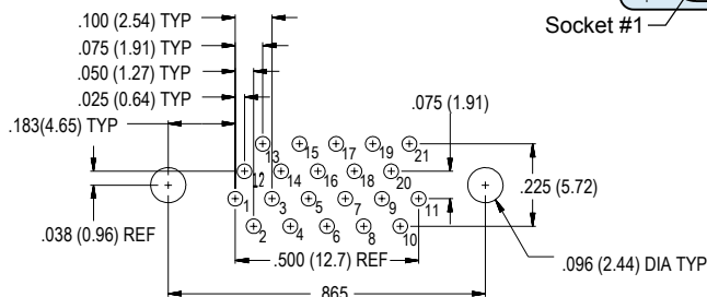
21 SOCKET M83513/31-C
