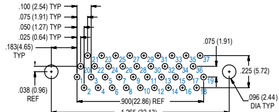
37 SOCKET
