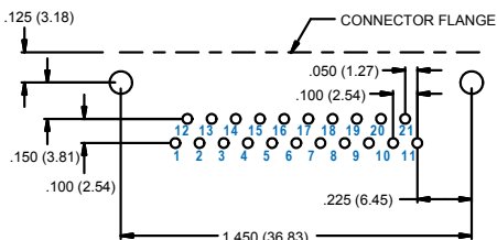
21 SOCKET M83513/19-C
