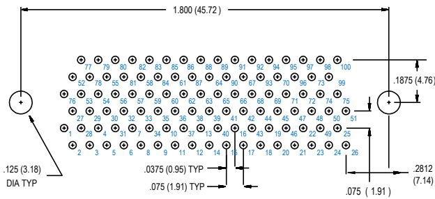
100 SOCKET
