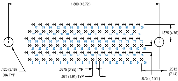
100 SOCKET
