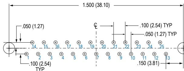
25 SOCKET M83513/25-D
