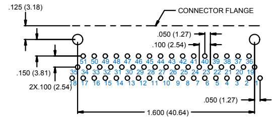
51 PIN M83513/17-G
