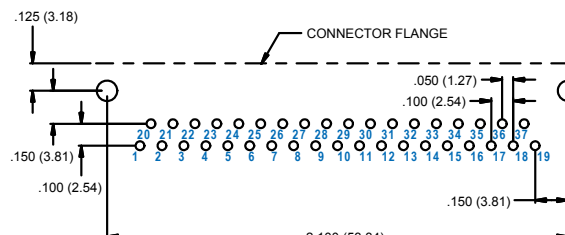
37 SOCKET M83513/19-F
