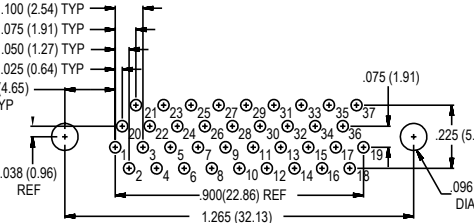
37 SOCKET
