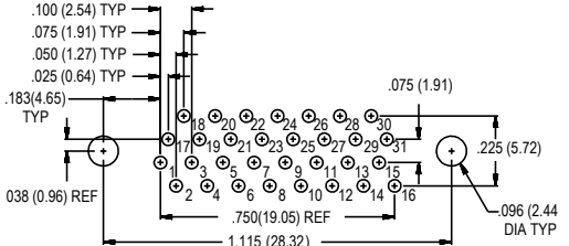
31 SOCKET
