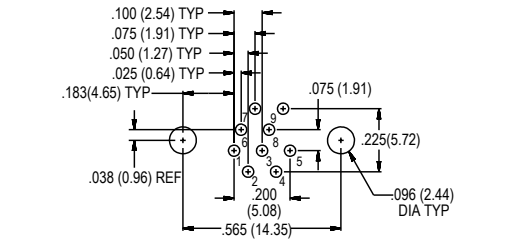
9 SOCKET
