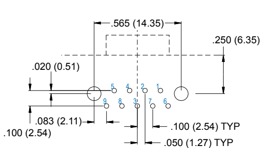
9 Socket
