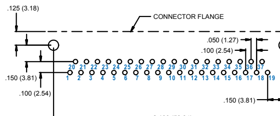
37 SOCKET M83513/19-F
