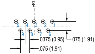
9 SOCKET
