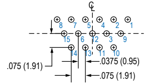
15 SOCKET
