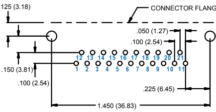
21 SOCKET M83513/19-C
