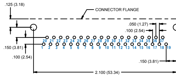
37 SOCKET M83513/19-F
