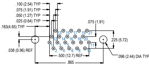
21 SOCKET
