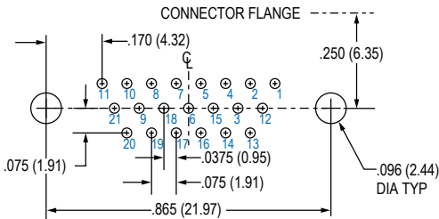
21 SOCKET
