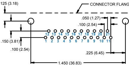
21 SOCKET M83513/19-C
