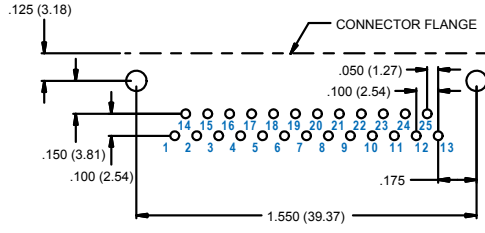
25 SOCKET M83513/19-D
