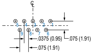
9 SOCKET
