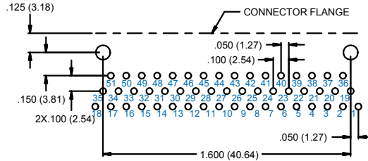
51 PIN M83513/17-G
