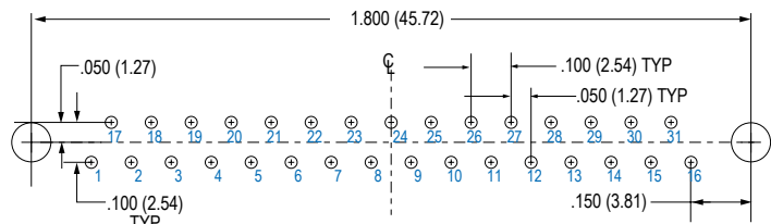
31 SOCKET
