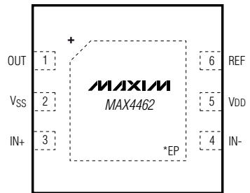
TDFN
