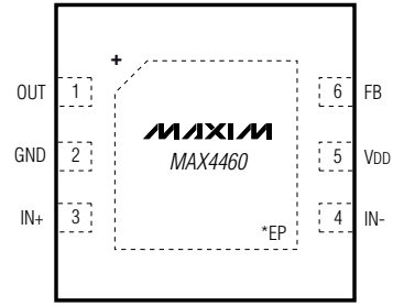
TDFN
