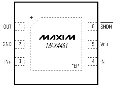
TDFN
