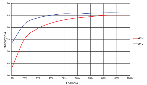
NCS12S4815C
