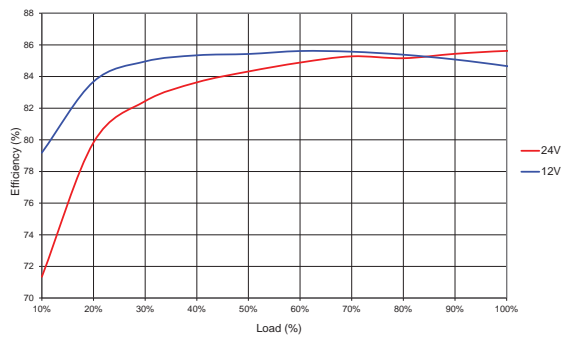
NCS12S4803C
