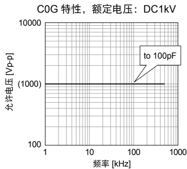
正弦频率 VS 容许电压
