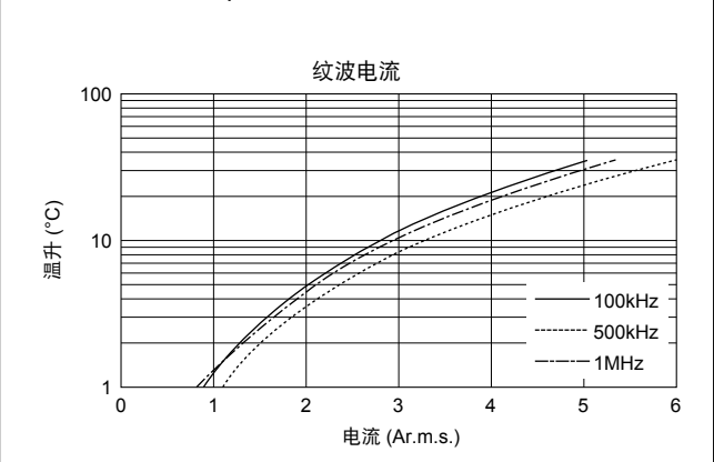
[与纹波电流相比，片状多层陶瓷电容器温升（热生成）示例] 示例：R 特性10μF，额定电压：DC10V
